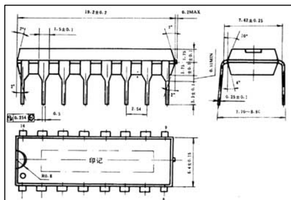
封装外形图
