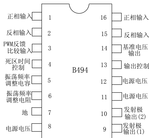
管脚排列图
